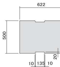
■平面図
