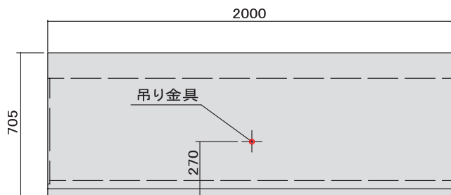
■側面図
