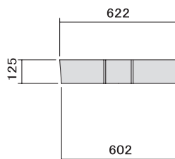
■断面図(車道用)
