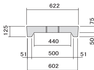
■断面図(歩道用)
