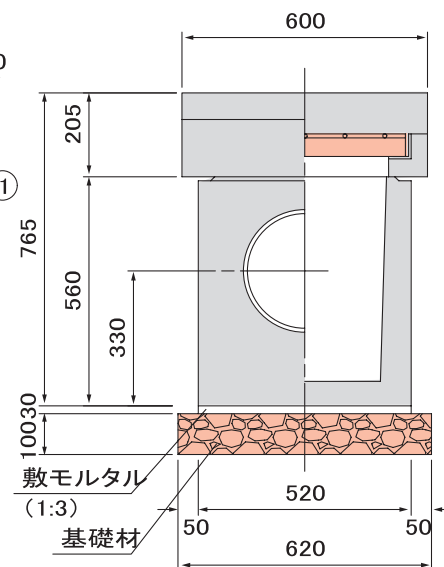
■縦断面図
