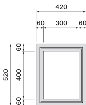
■①—①断面図
