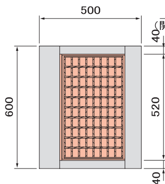
■平面図
