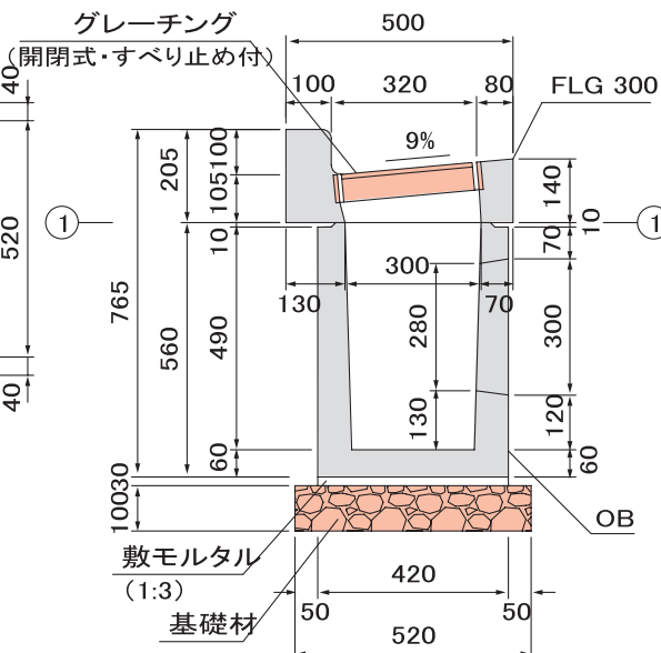
■横断面図
