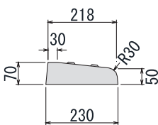
■ 端部正面図
