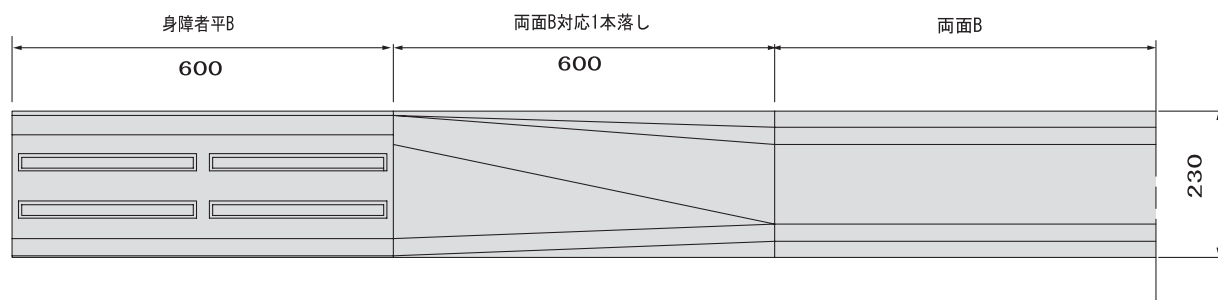
■側面図
